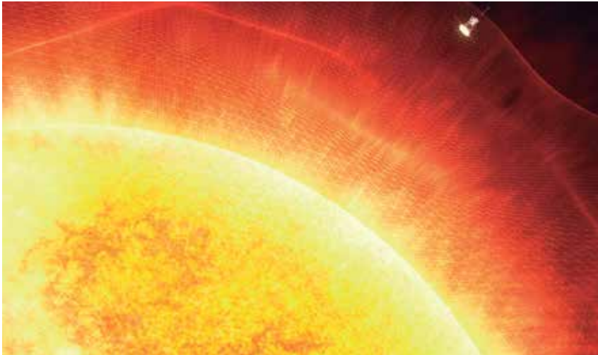
La NASA revela representaciones gráficas de las imágenes inéditas captadas del Sol que aclaran los misterios del clima espacial. NASA / JOHNS HOPKINS APL / BEN SMITH 16/JUL
