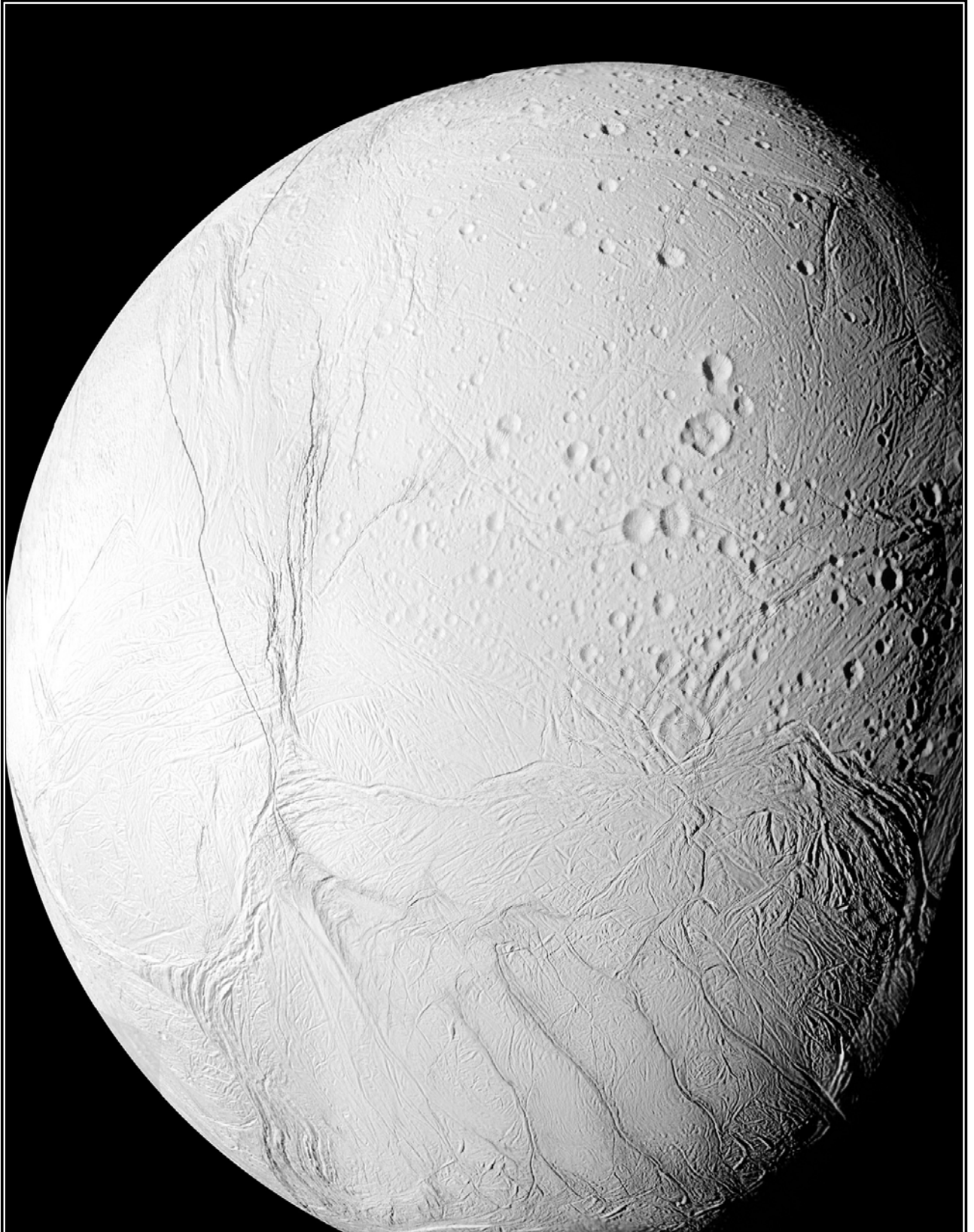
La sonda Cassini de la agencia espacial estadounidense NASA descubrió reservas de agua en la pequeña y misteriosa luna Encelado, de Saturno. La imagen muestra una de las caras del satélite ■ Ap
